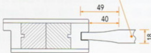
SEZIONE ANTA CON PANNELLETTO BUGNATO
