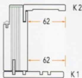
TELAIO R02
