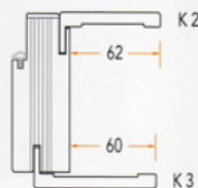
TELAIO R02
